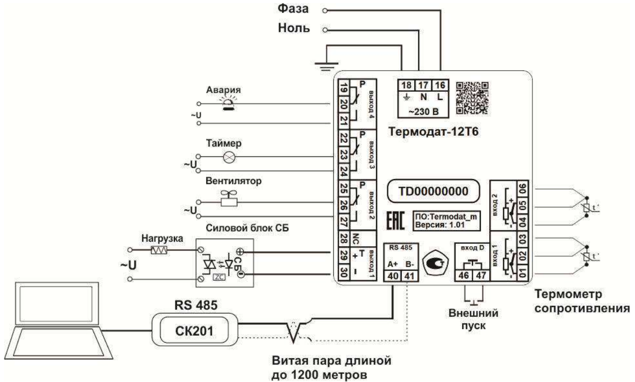
Рисунок 7 – Схема подключения прибора.
